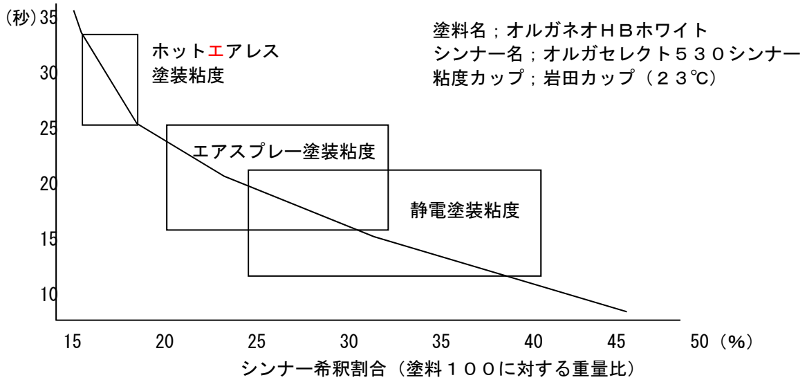
図-2 希釈率、粘度曲線
