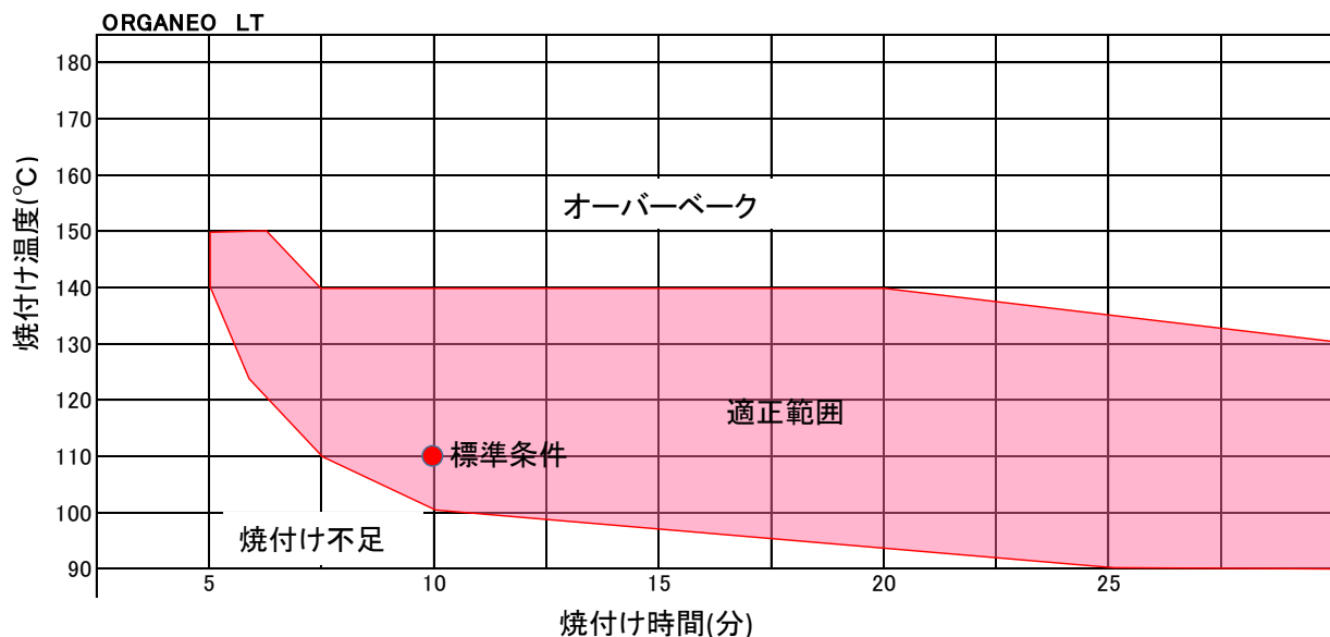
図-1 オルガネオLT、エコLTの焼付け温度と時間の関係（被塗物のキープ条件）
