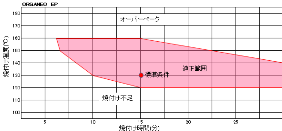
図-1 オルガネオEPの焼付け温度と時間の関係（被塗物のキープ条件）
