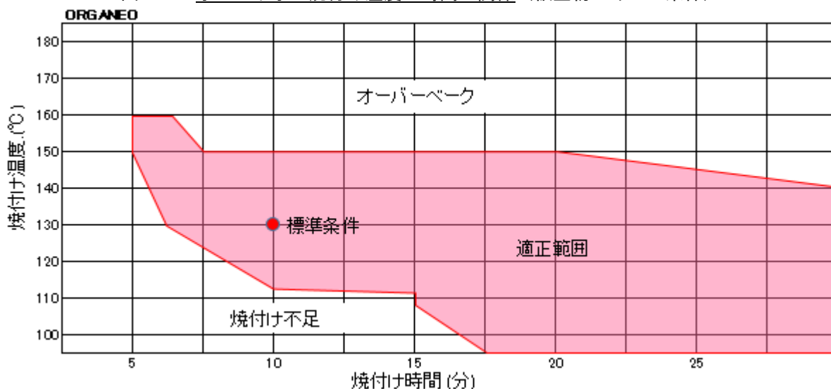
図-1 オルガネオの焼付け温度と時間の関係（被塗物のキープ条件）
