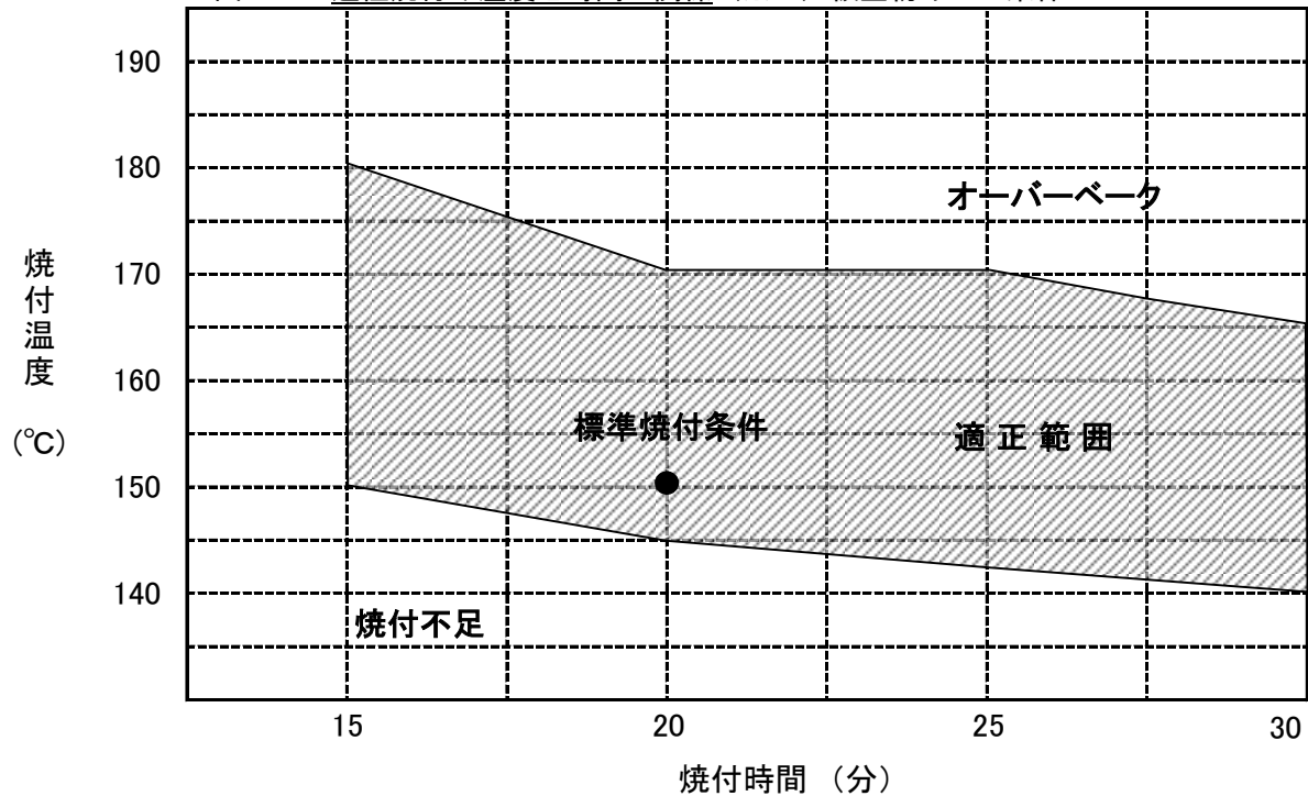
図-1 適性焼付け温度と時間の関係 (※1) 被塗物キープ条件
