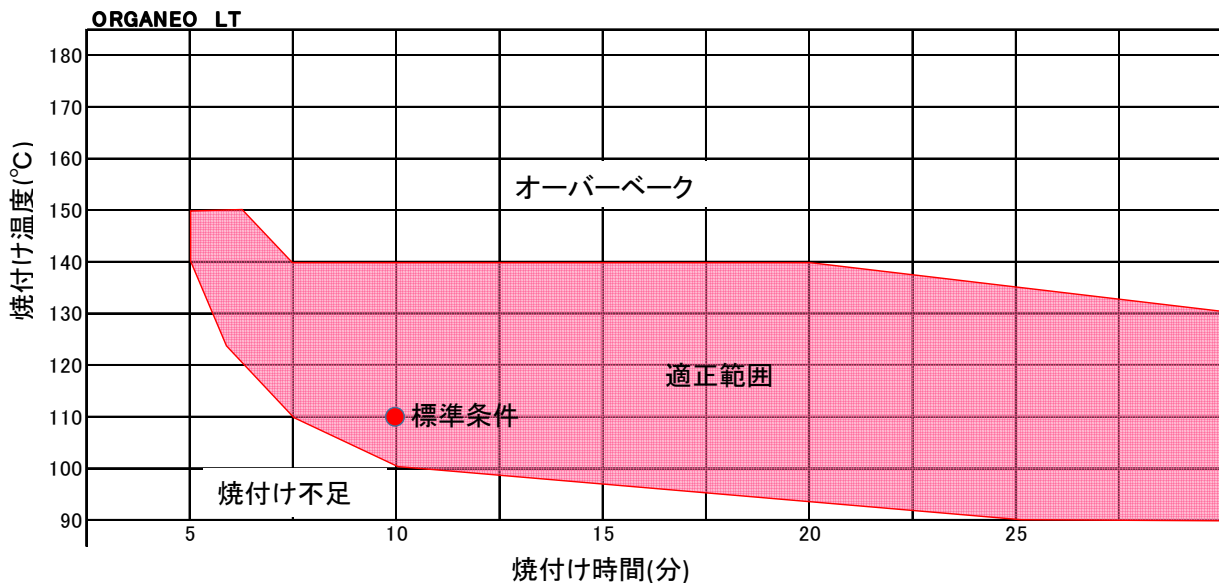
図-1 オルガネオLTの焼付け温度と時間の関係 （被塗物のキープ条件）
