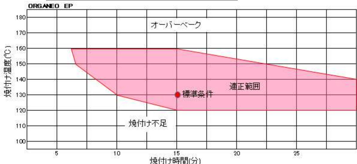
図-1 オルガネオEP、エコEPの焼付け温度と時間の関係（被塗物のキープ条件）
