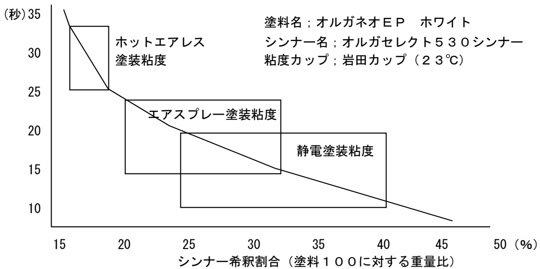
図-2 希釈率、粘度曲線
