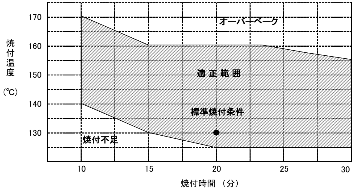
図-1 適性焼付け温度と時間の関係 (※1) 被塗物キープ条件
