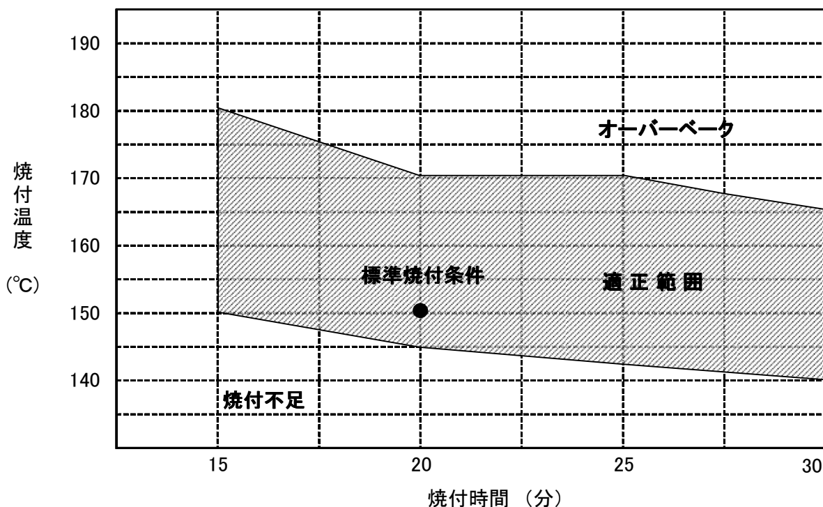
図ー1 適性焼付け温度と時間の関係（※1）被塗物キープ条件
